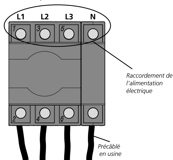
Bloc coupe-circuit.
