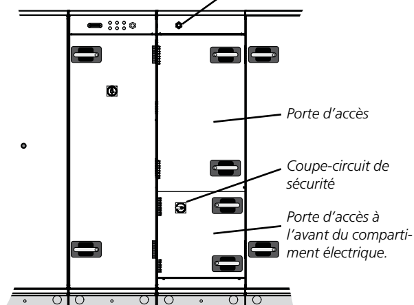
Bloc coupe-circuit.
