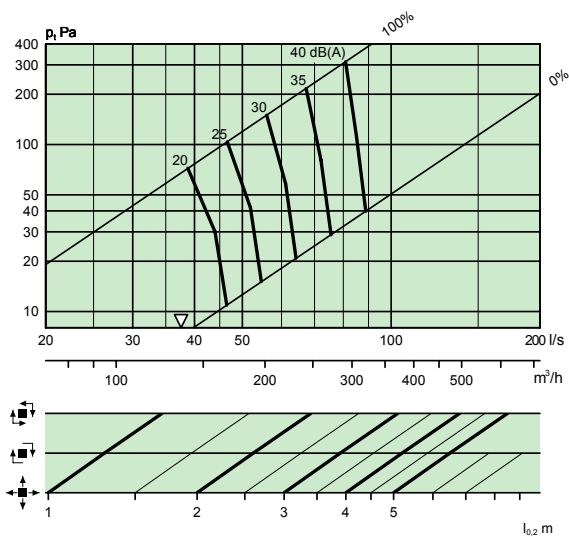
COLIBRI CC 200-500 + ALS 160-200 – 1 Schritte
