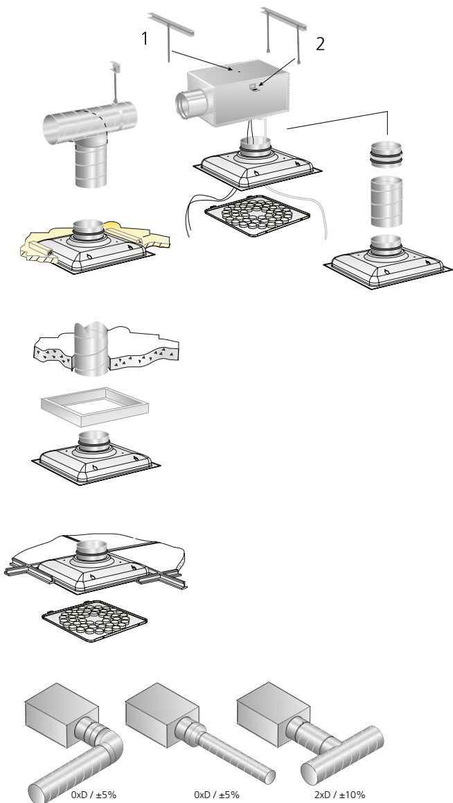
Abbildung 2. Montage.
