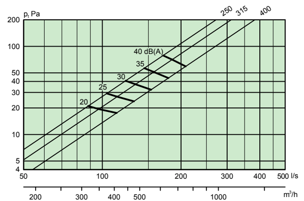
COLIBRI CR 250-600, 315-600 und 400-600 – Abluft
