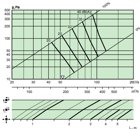
COLIBRI CC 250-600 + ALS 160-250 – 2 Schritte
