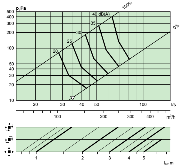
COLIBRI CC 200-500 + ALS 125-200 – 2 Schritte
