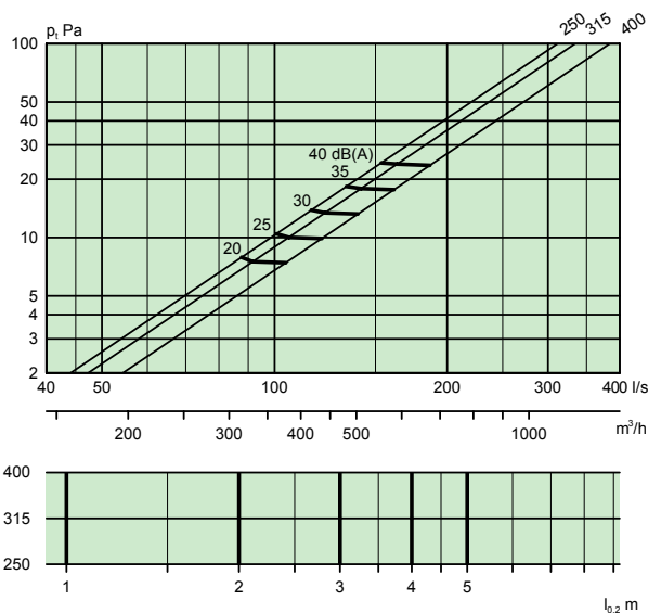
COLIBRI CR 250-600, 315-600 und 400-600 – Zuluft
