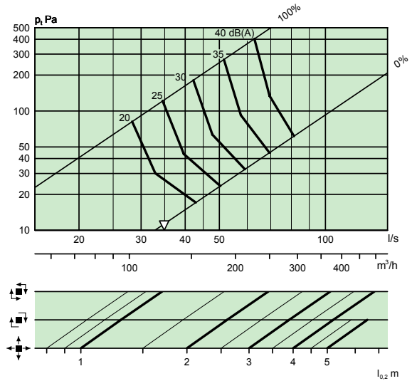
COLIBRI CC 200-600 + ALS 125-200 – 2 Schritte
