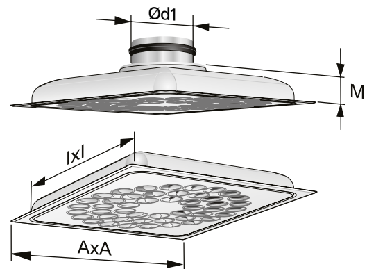
Abbildung 5. COLIBRI Ceiling
