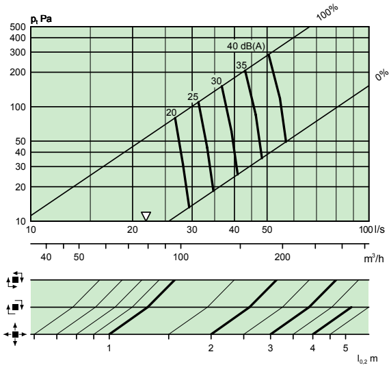
COLIBRI CC 160-400 + ALS 125-160 – 1 Schritte
