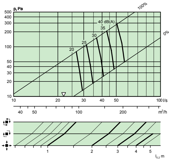
COLIBRI CC 160-600 + ALS 125-160 – 1 Schritte
