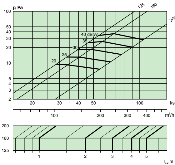
COLIBRI CR 125-400, 160-400 und 200-500 – Zuluft
