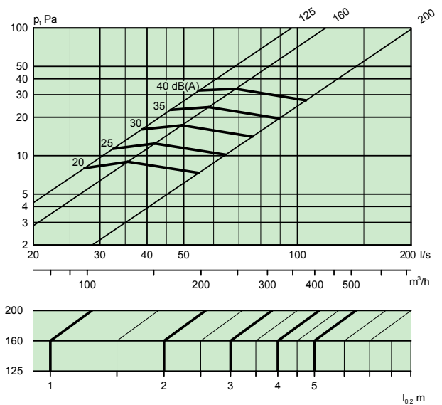
COLIBRI CR 125-600, 160-600 und 200-600 – Zuluft
