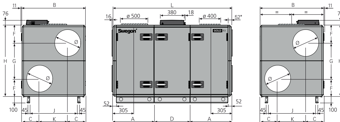
GOLD 007/008, gedeeld ontwerp
