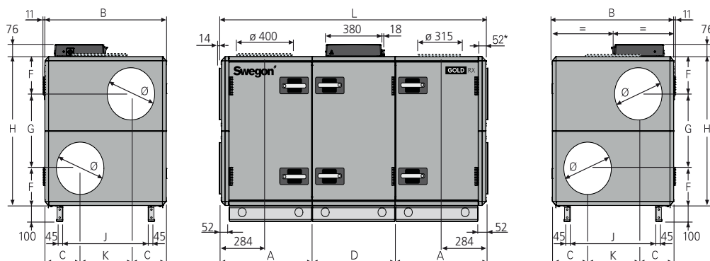
GOLD 007/008, gedeeld ontwerp
