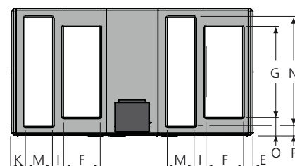
Bovenaanzicht. Toont de kanaalaansluitingen van de luchtbehandelingsunit voor toevoerluchtventilator rechtsonder en linksboven
