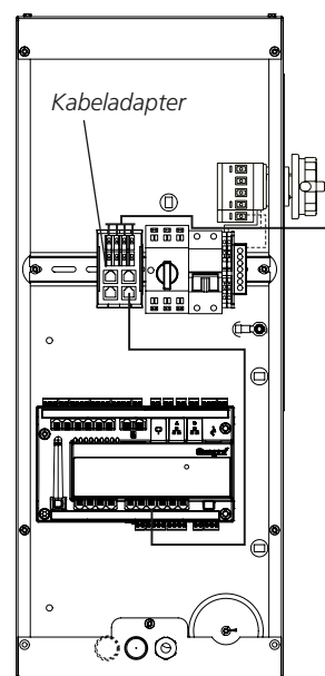
GOLD SD med styreenhed (tilluft)
