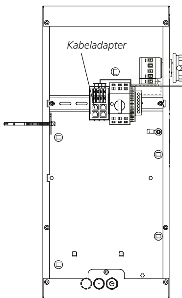
GOLD SD uden styreenhed (fraluft)
