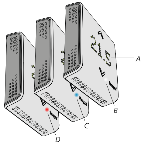
Kuva 3. WISE RTA, LED-numerot ja merkkivalot. A. Vihreät LEDit näyttävät asetusarvon. B. Valkoinen valo pariliitostilassa C. Sininen valo osoittaa jäädytystarpeen D. Punainen valo osoittaa lämmitystarpeen
