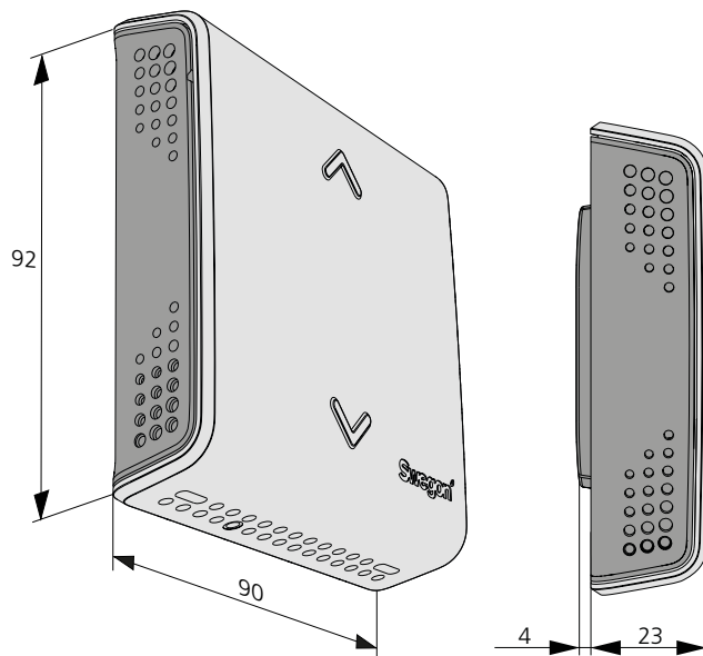
Kuva 5. Mitat, WISE RTA.
