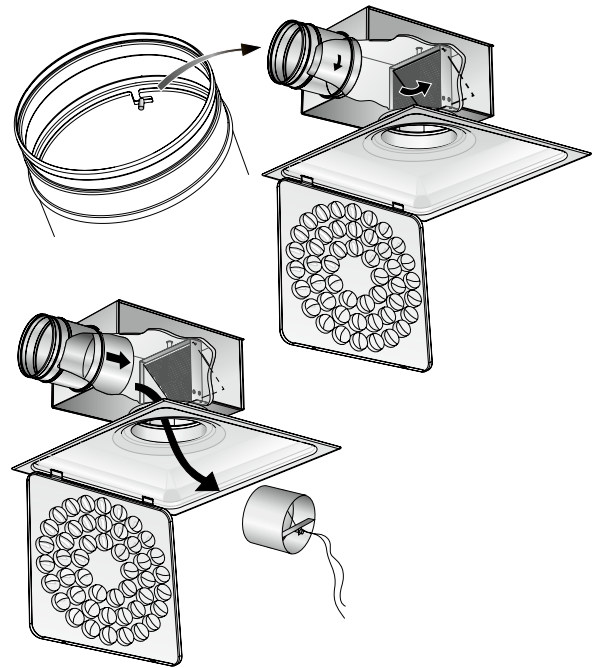
Abb. 3. Demontage von Klappen bei Verwendung des Anschlusskastens REACT ALS und ALS.
