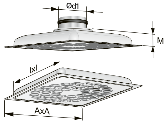
Abb. 4. COLIBRI Ceiling VF.
