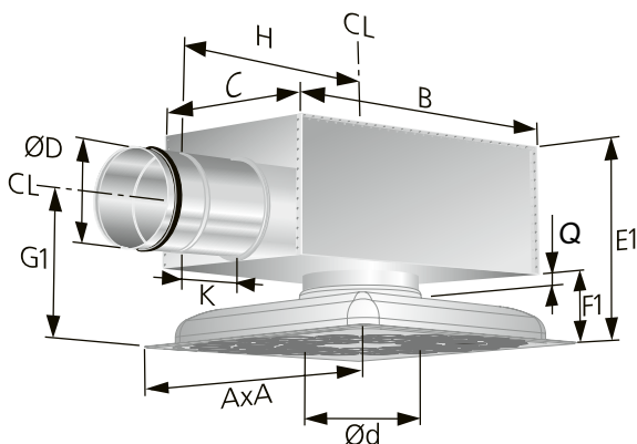
Abb. 5. COLIBRI Ceiling VF mit Anschlusskasten REACT ALS oder ALS. CL = Mittellinie.
