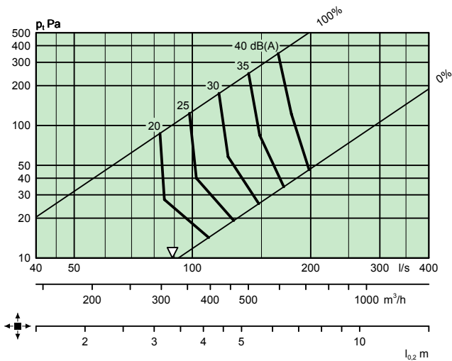
CKP 250 + ALS 200-250
