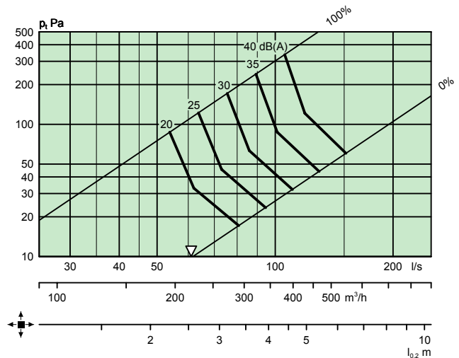
CKP 200 + ALS 160-200
