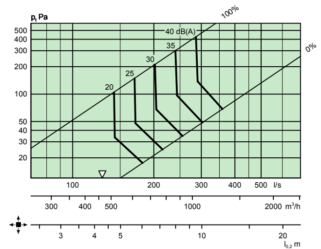
CDK 315 + ALS 250-315
