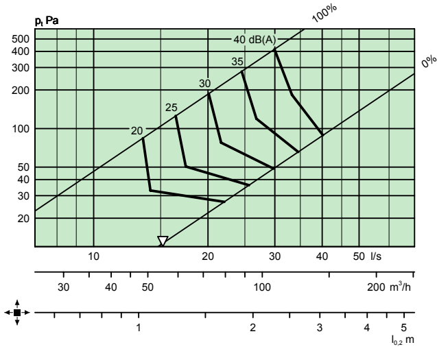
CKP 100 + ALS 80-100
