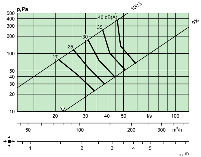
CKP 125 + ALS 100-125
