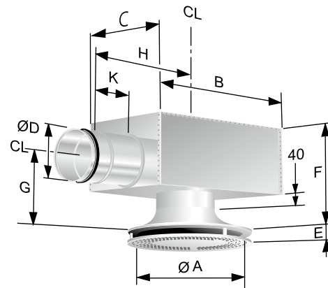
Abbildung 3. CDK/CKP + ALS
