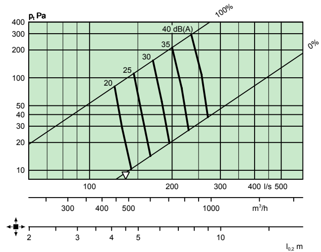
CKP 315-ALS 250-315
